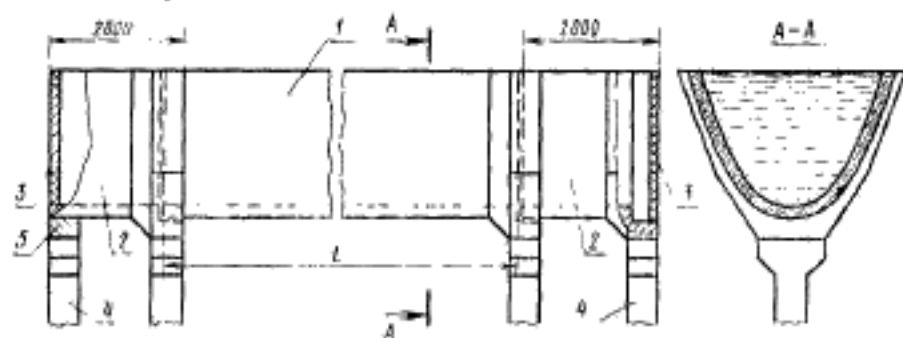
1—испытуемый лоток; 2—укороченный лоток (2 шт.); 3—заглушки; 4—опоры лотков; 5—прокладка.
